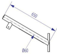
CẢN ĐÈN / ARM CD-T18-G5
