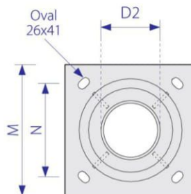
ĐỂ CỘT / BASE PLATE
