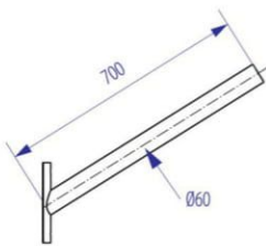
CẢN ĐÈN / ARM CD-T18-L700
