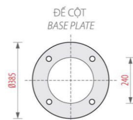
ĐỂ CỘT BASE PLATE Khung móng Anchor bolts 4/M16 x 500
