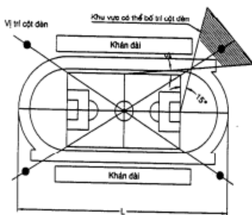
c. Sân đa chức năng - Phương án sử dụng 04 cột đèn
