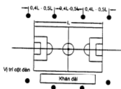
b. Sân bóng đá - Phương án sử dụng 08 cột đèn
