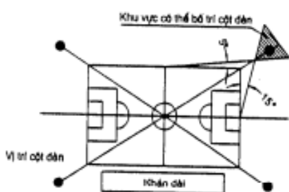
a. Sân bóng đá - Phương án sử dụng 04 cột đèn
