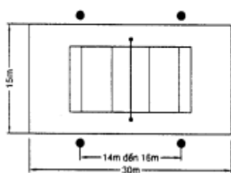
a. Phương án sử dụng 04 cột đèn : Sân thi đấu - Luyện tập
