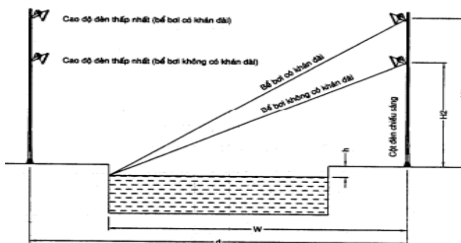
Hình 9: Cao độ đặt đèn chiếu sáng bể bơi ngoài trời
