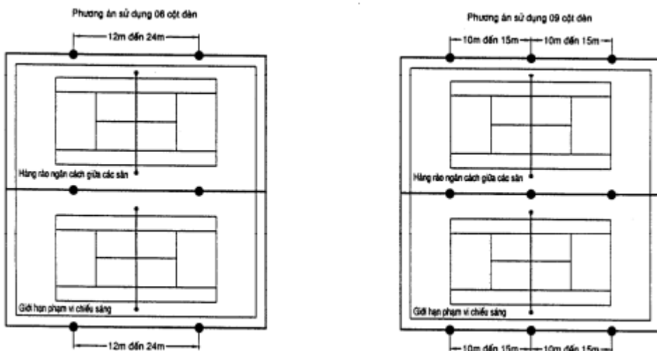
Hình 23: Bố trí cột đèn chiếu sáng sân quần vợt có hàng rào ngăn cách
