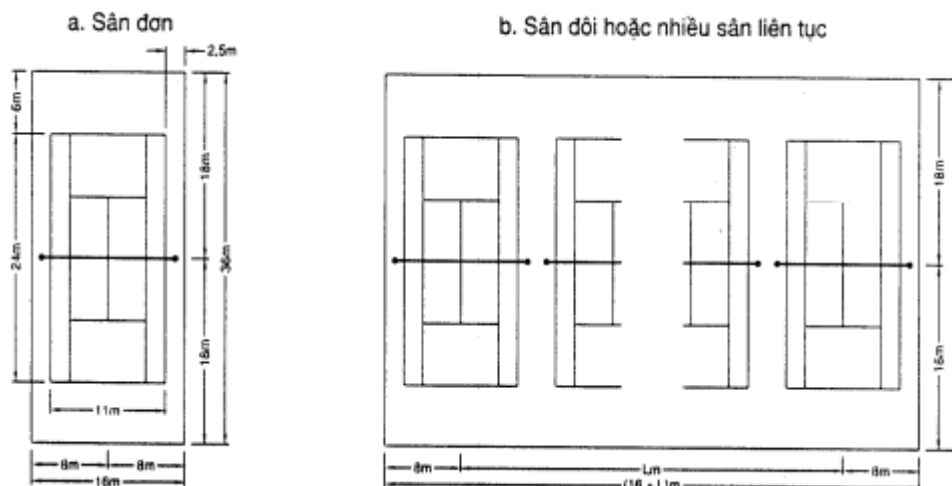
Hình 5: Diện tích đo đạc và tính toán chiếu sáng sân quần vợt
