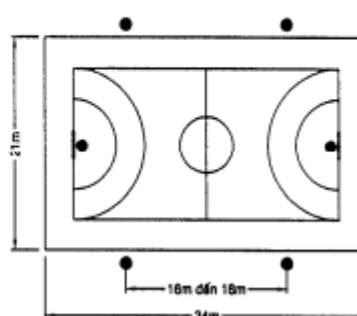
b. Phương án sử dụng 04 cột đèn : Chỉ áp dụng đối với sân luyện tập
