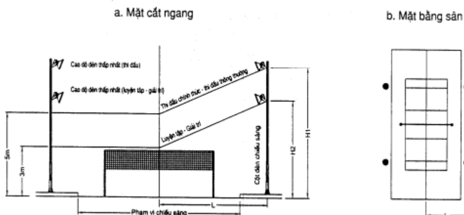
Hình 8: Cao độ đặt đèn và khoảng cách chiếu sáng sân Bóng chuyền - Bóng rổ - Cầu lông
