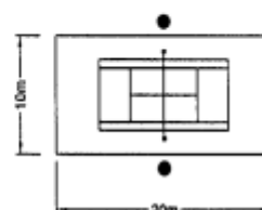
b. Phương án sử dụng 02 cột đèn : Chỉ áp dụng đối với sân luyện tập
