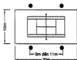
a. Phương án sử dụng 04 cột đèn : Sân thi đấu - Luyện tập
