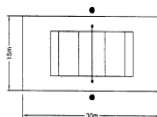
b. Phương án sử dụng 02 cột đèn : Chỉ áp dụng đối với sân luyện tập
