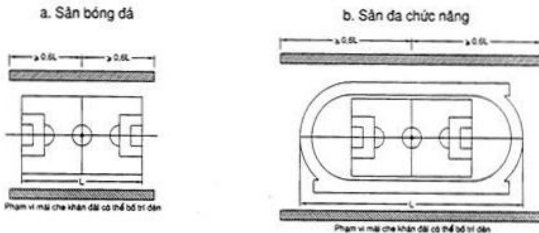
Hình 21 : Bố trí đèn chiếu sáng trên mái che khán đài
