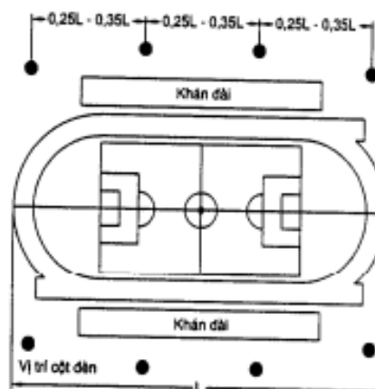
d. Sân đa chức năng - Phương án sử dụng 08 cột đèn
