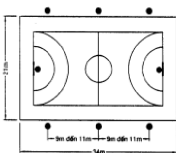
a. Phương án sử dụng 06 cột đèn : Sân thi đấu - Luyện tập
