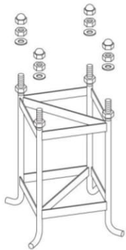
ĐỂ CỘT BASE PLATE
