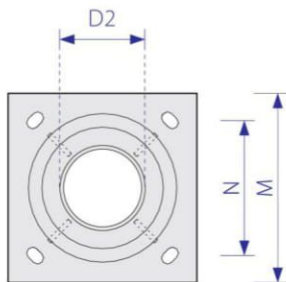
ĐỂ CỘT BASE PLATE
